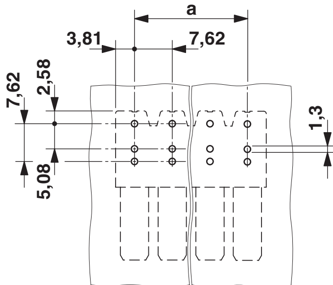
Bohrplan/Lötpadgeometrie
