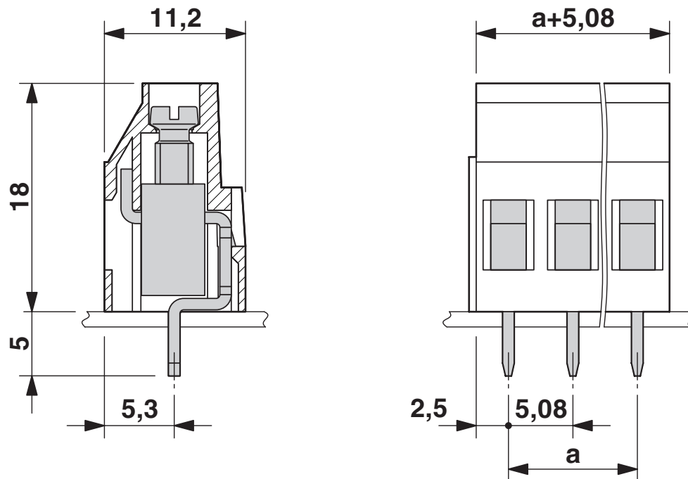
Maßzeichnung
