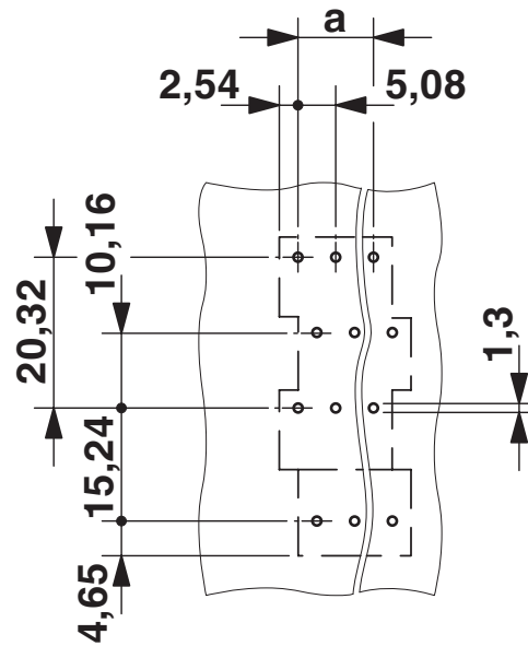
Bohrplan/Lötpadgeometrie
