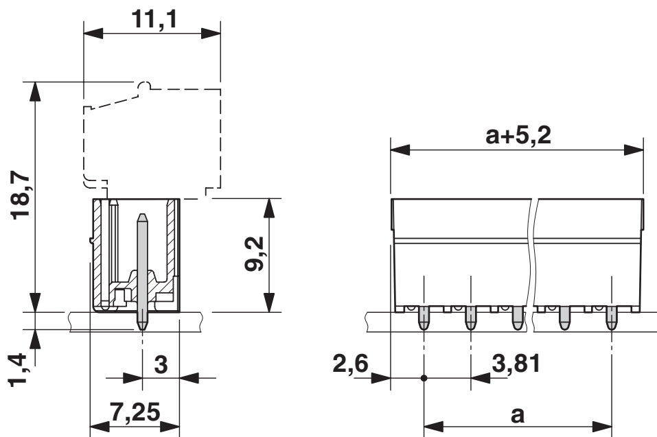
Maßzeichnung
