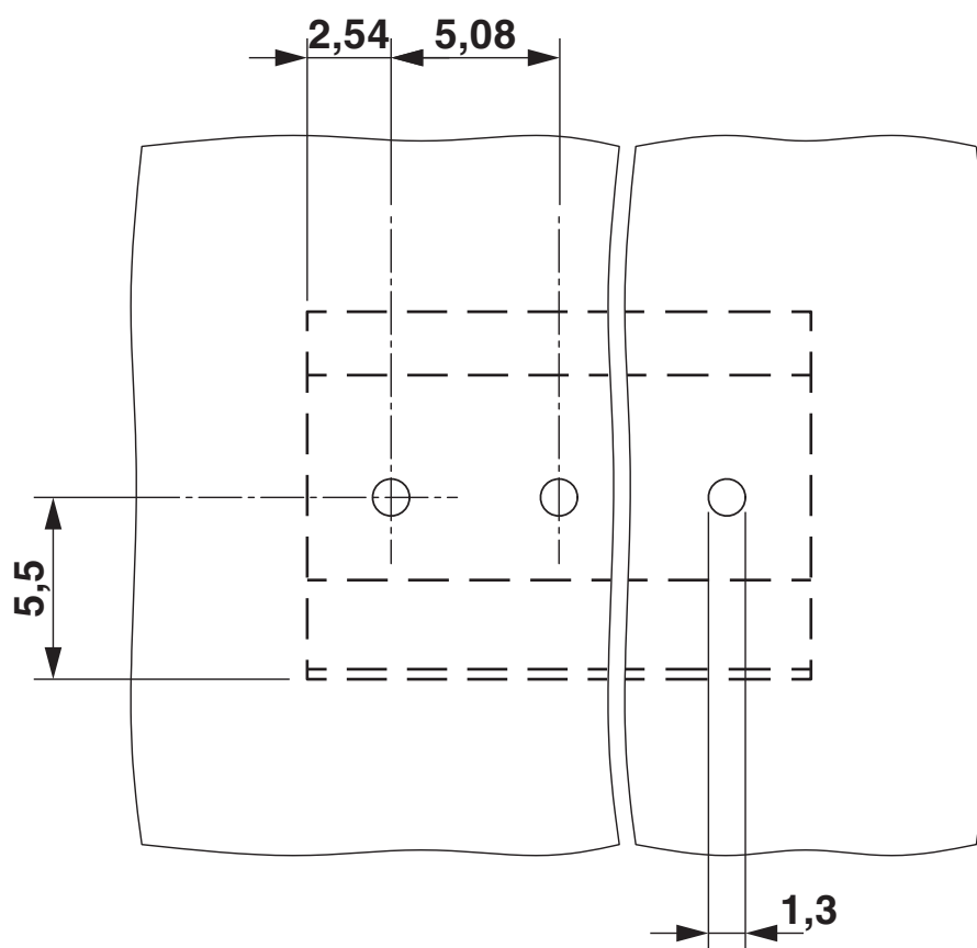
Bohrplan/Lötpadgeometrie
