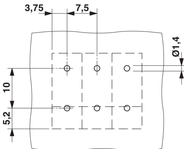
Bohrplan/Lötpadgeometrie
