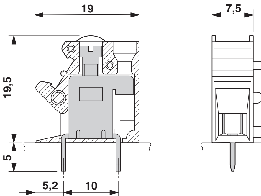
Maßzeichnung
