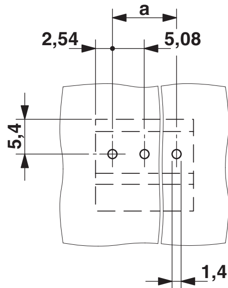
Bohrplan/Lötpadgeometrie
