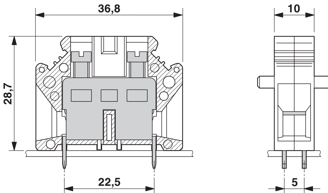
Maßzeichnung
