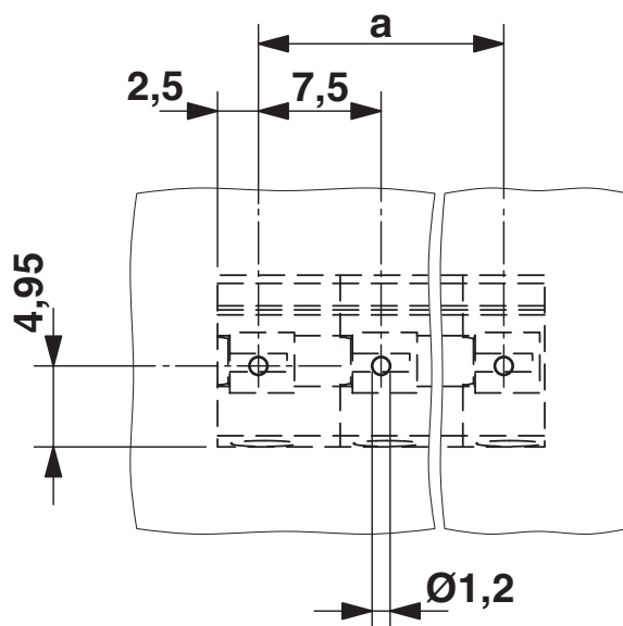
Bohrplan/Lötpadgeometrie
