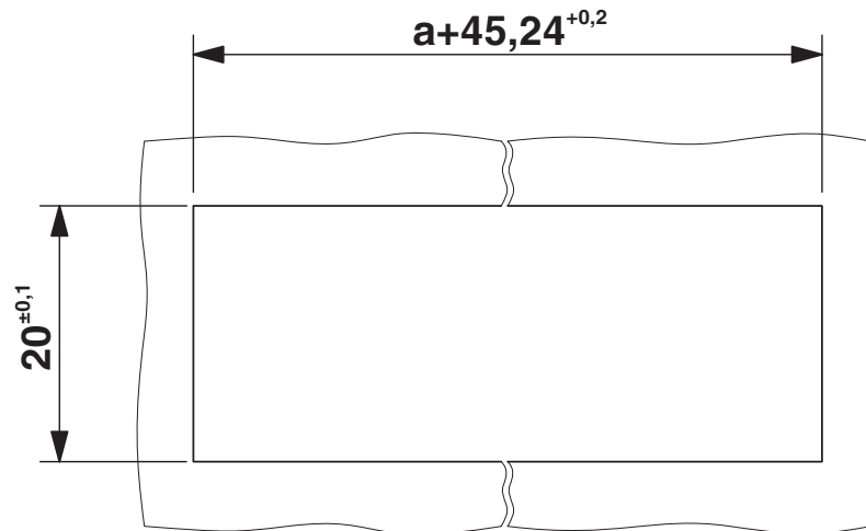
Maßzeichnung
