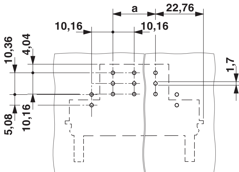
Bohrplan/Lötpadgeometrie
