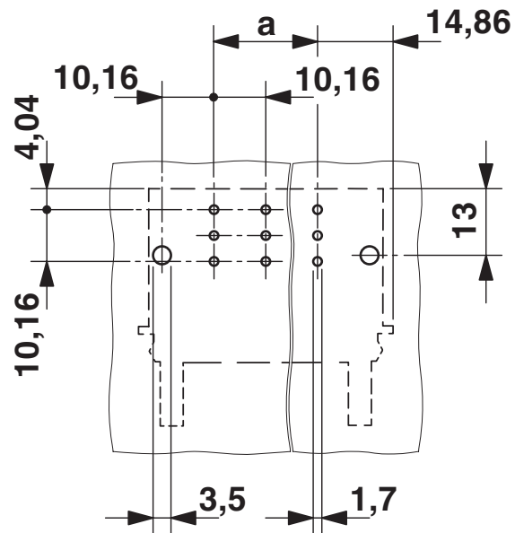
Bohrplan/Lötpadgeometrie
