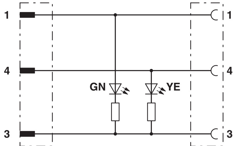
Schaltplan
