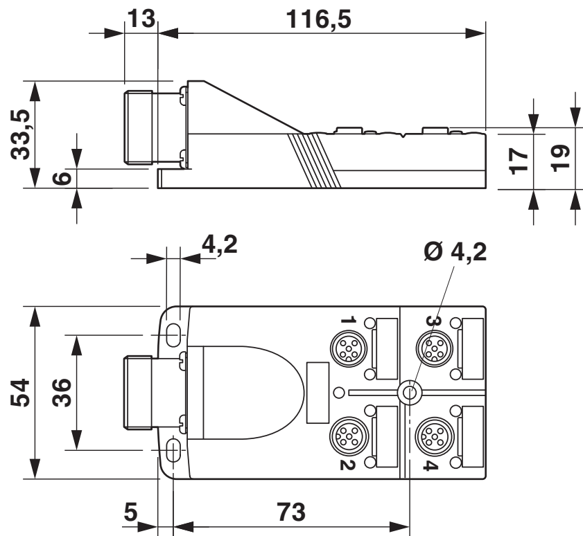
Maßzeichnung
