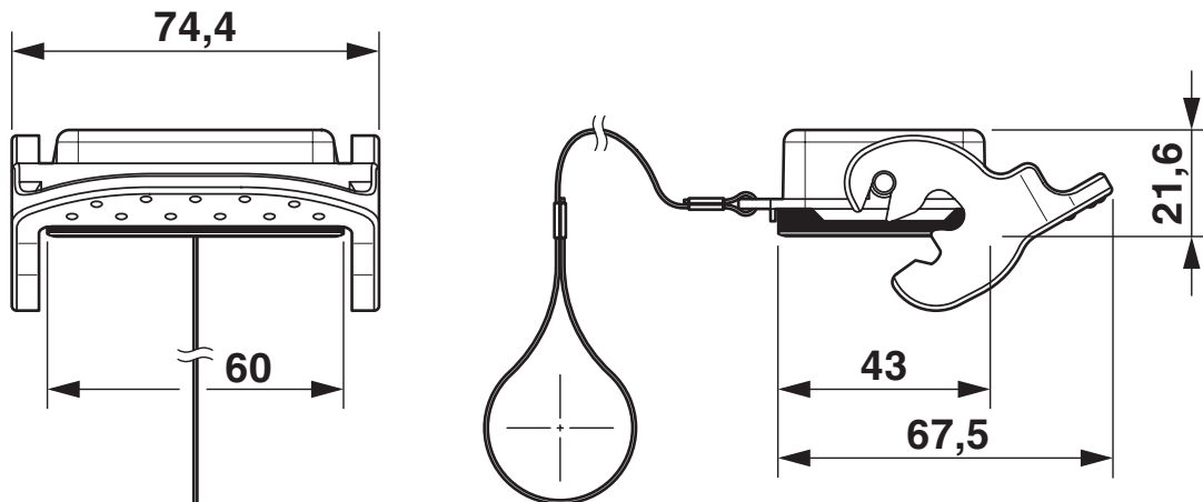
Maßzeichnung
