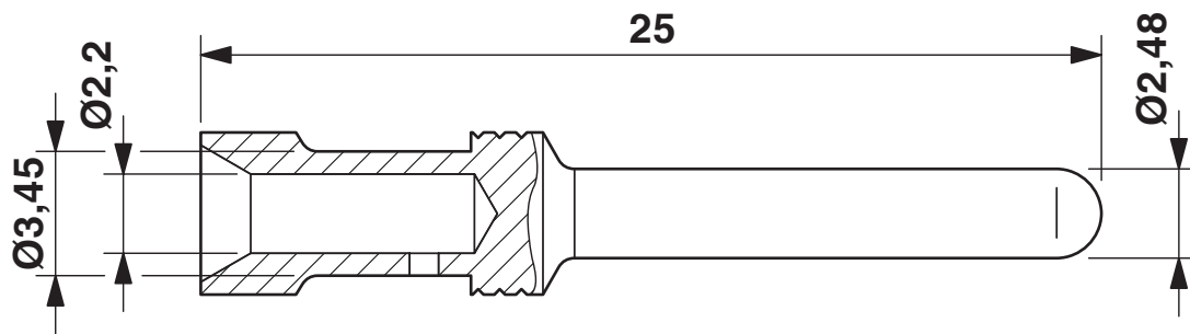
Maßzeichnung
