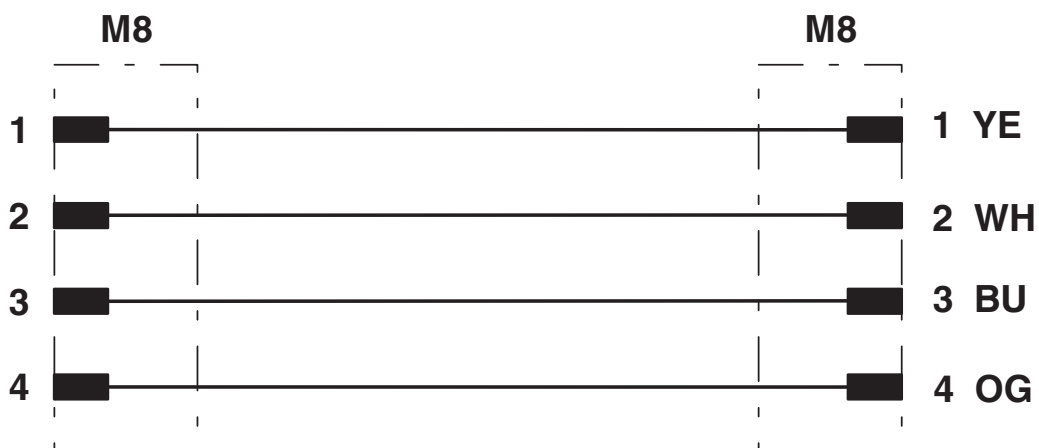
Kontaktbelegung der M8-Stecker
