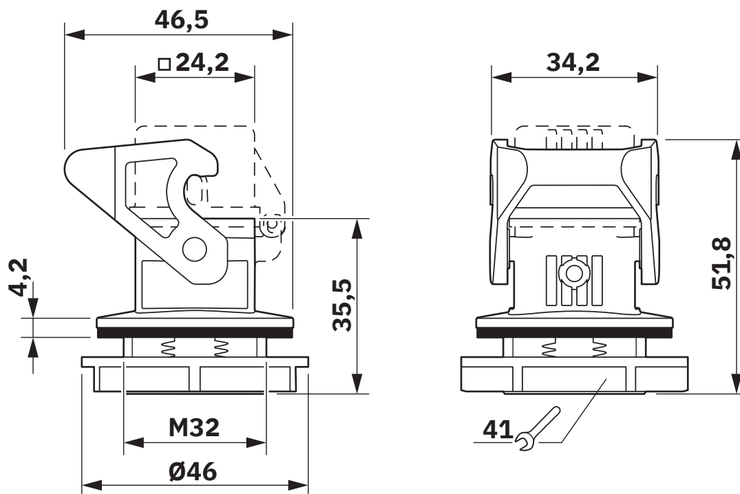
Maßzeichnung
