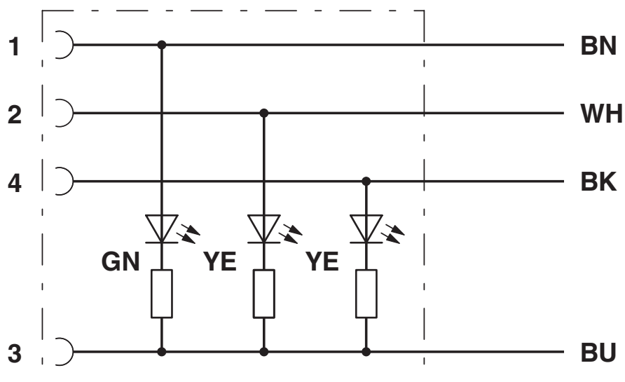
Kontaktbelegung der M12-Stecker / Buchsen mit LED
