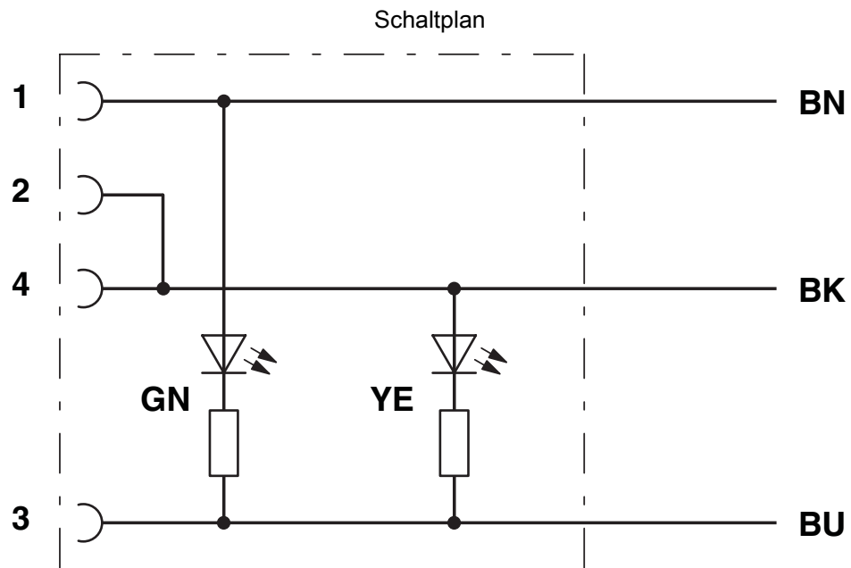
Kontaktbelegung der M12-Buchse mit LED, gebrückt
