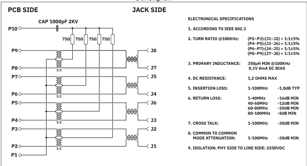
Schaltplan
