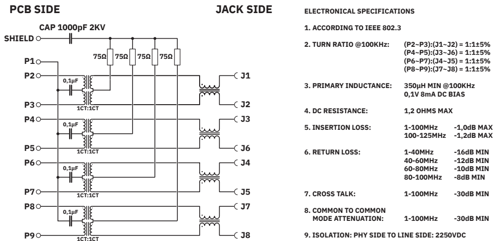
Schaltplan
