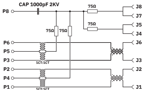
Schaltplan Jack Side
