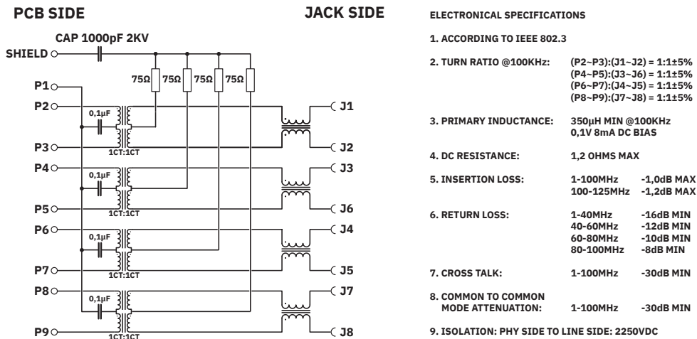
Schaltplan
