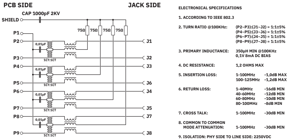
Schaltplan
