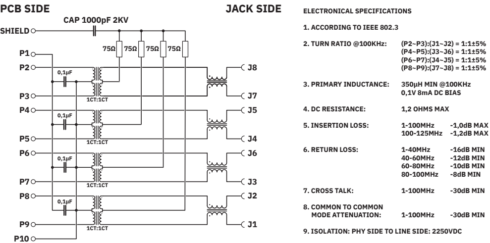
Schaltplan
