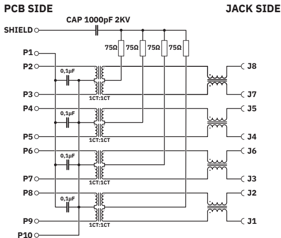
Schaltplan JACK SIDE
