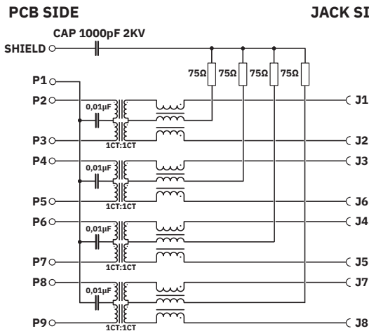
Schaltplan JACK SIDE
