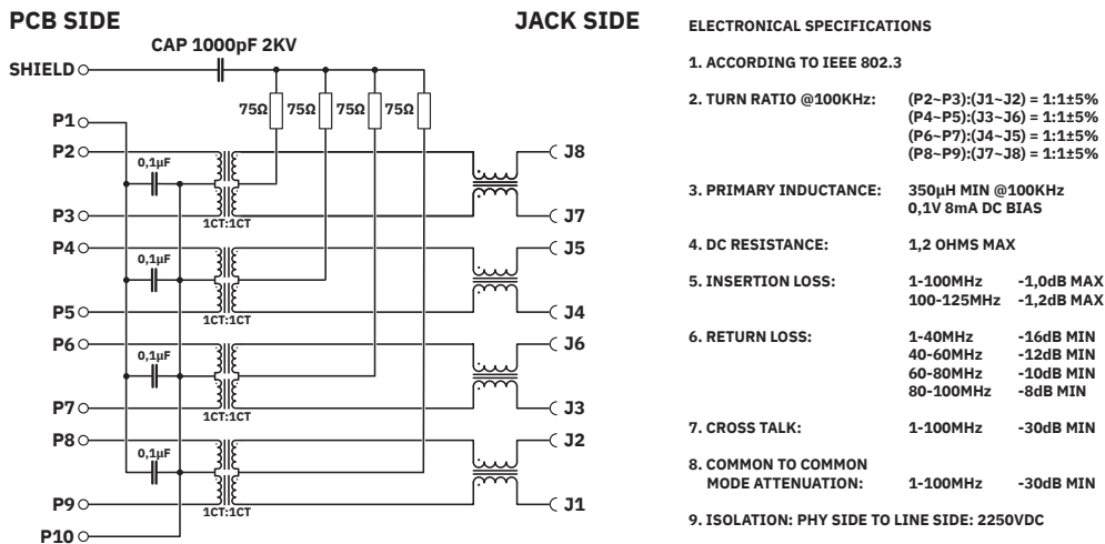
Schaltplan
