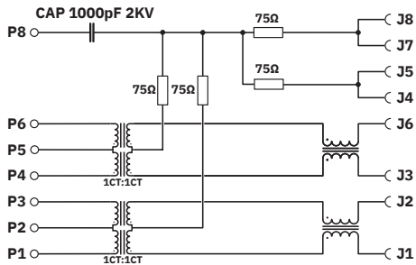
Schaltplan
