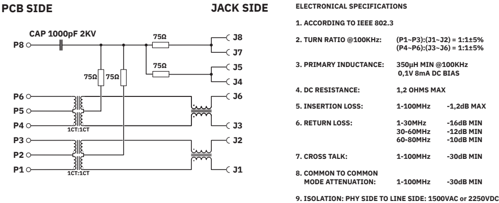
Schaltplan
