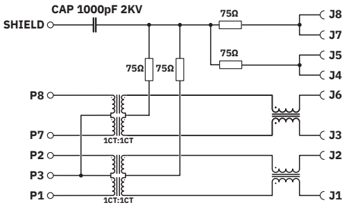
Schaltplan
