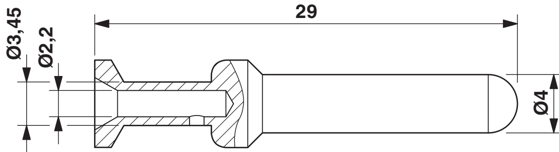
Maßzeichnung
