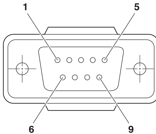
Schemazeichnung
