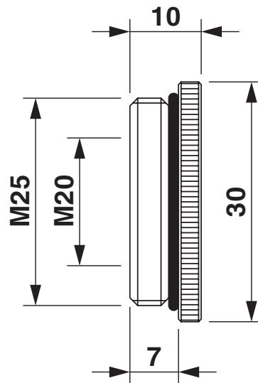
Maßzeichnung
