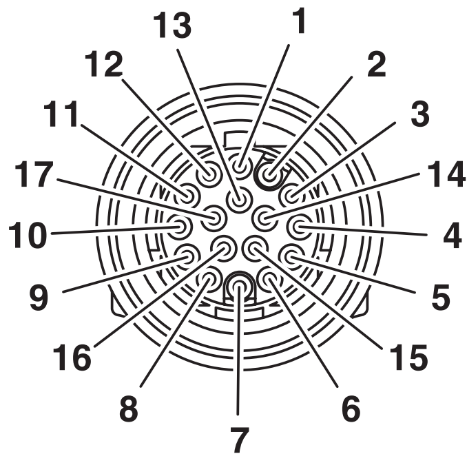
Schemazeichnung
