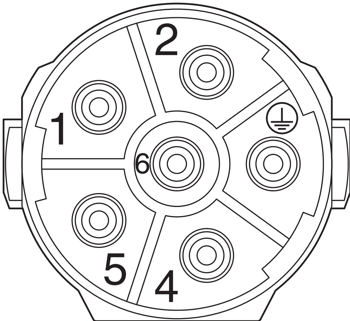
Schemazeichnung
