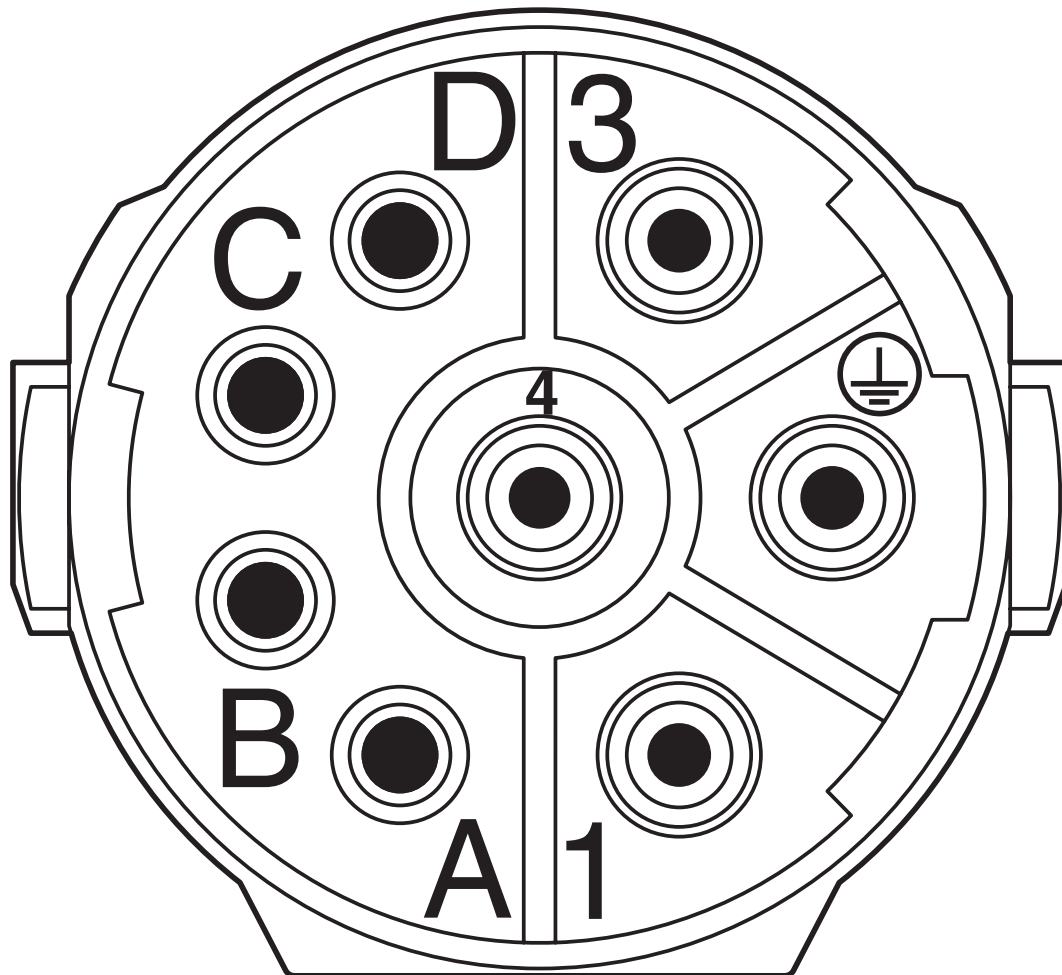
Schemazeichnung
