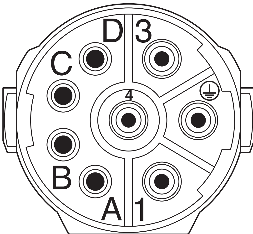
Schemazeichnung
