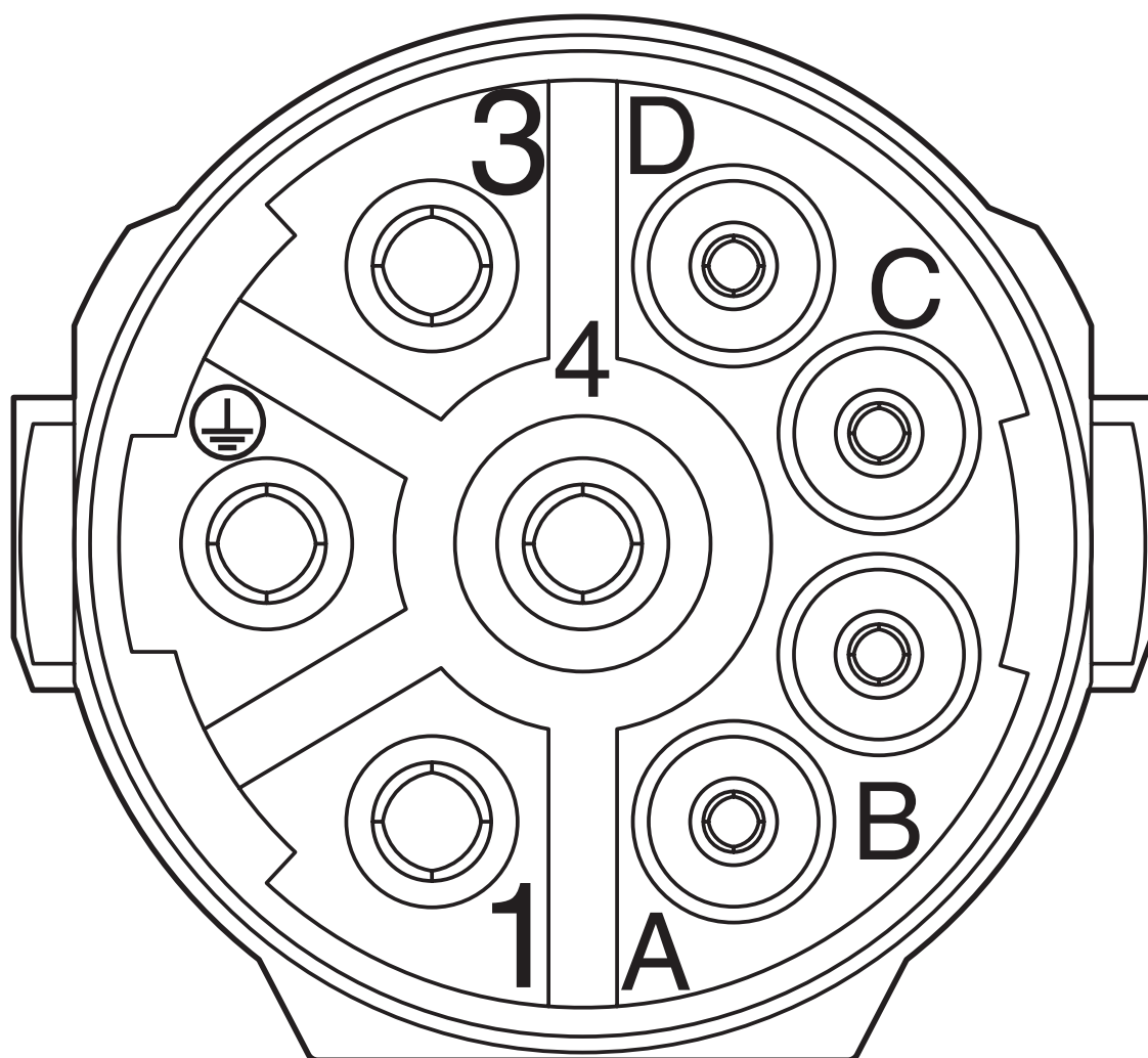
Schemazeichnung
