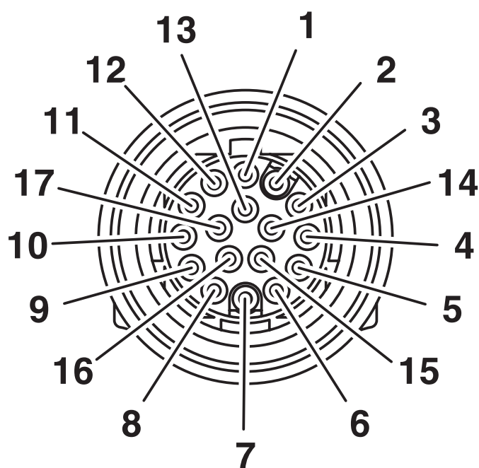
Schemazeichnung
