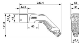
Infrastruktur-Ladestecker
