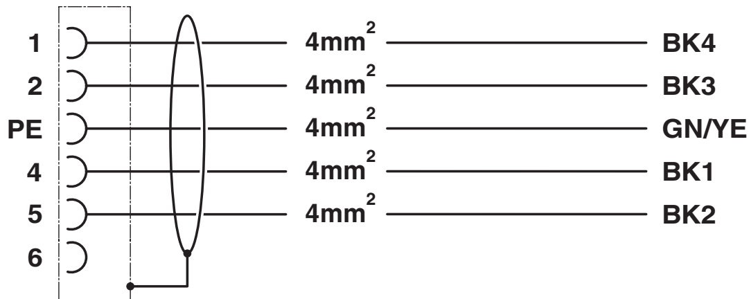
Schaltplan
