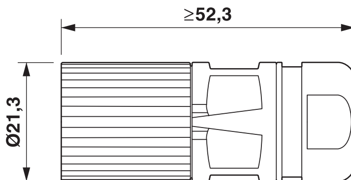
Maßzeichnung
