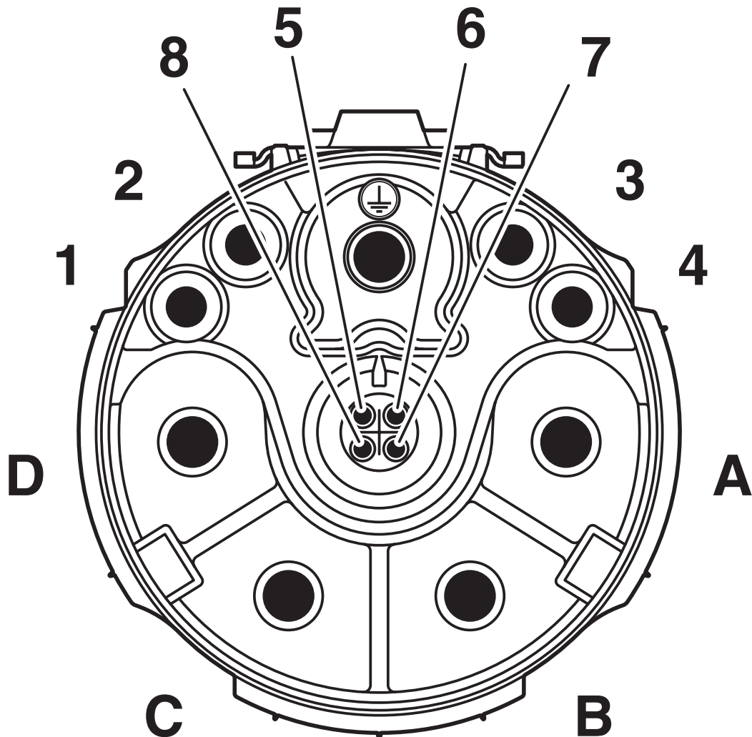
Schemazeichnung
