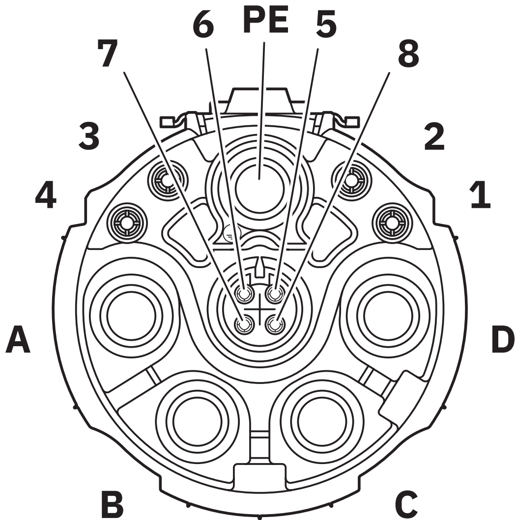
Schemazeichnung
