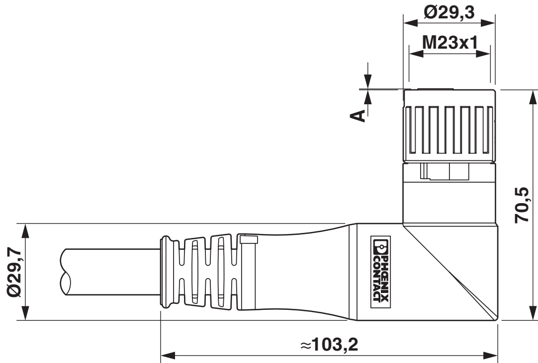
Maßzeichnung
