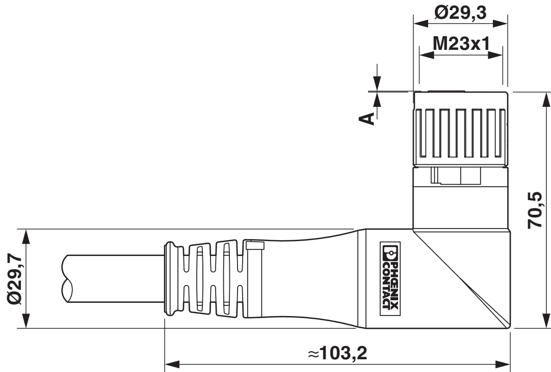
Maßzeichnung
