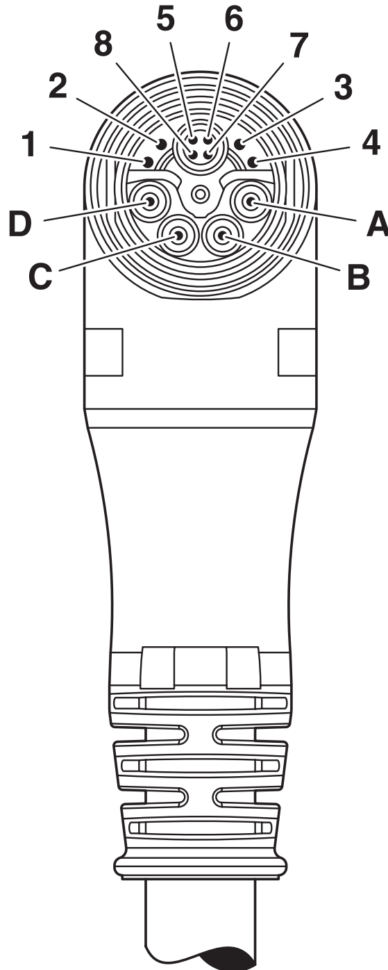
Schemazeichnung
