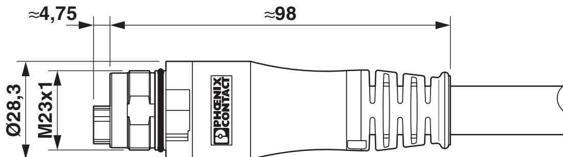
Maßzeichnung
