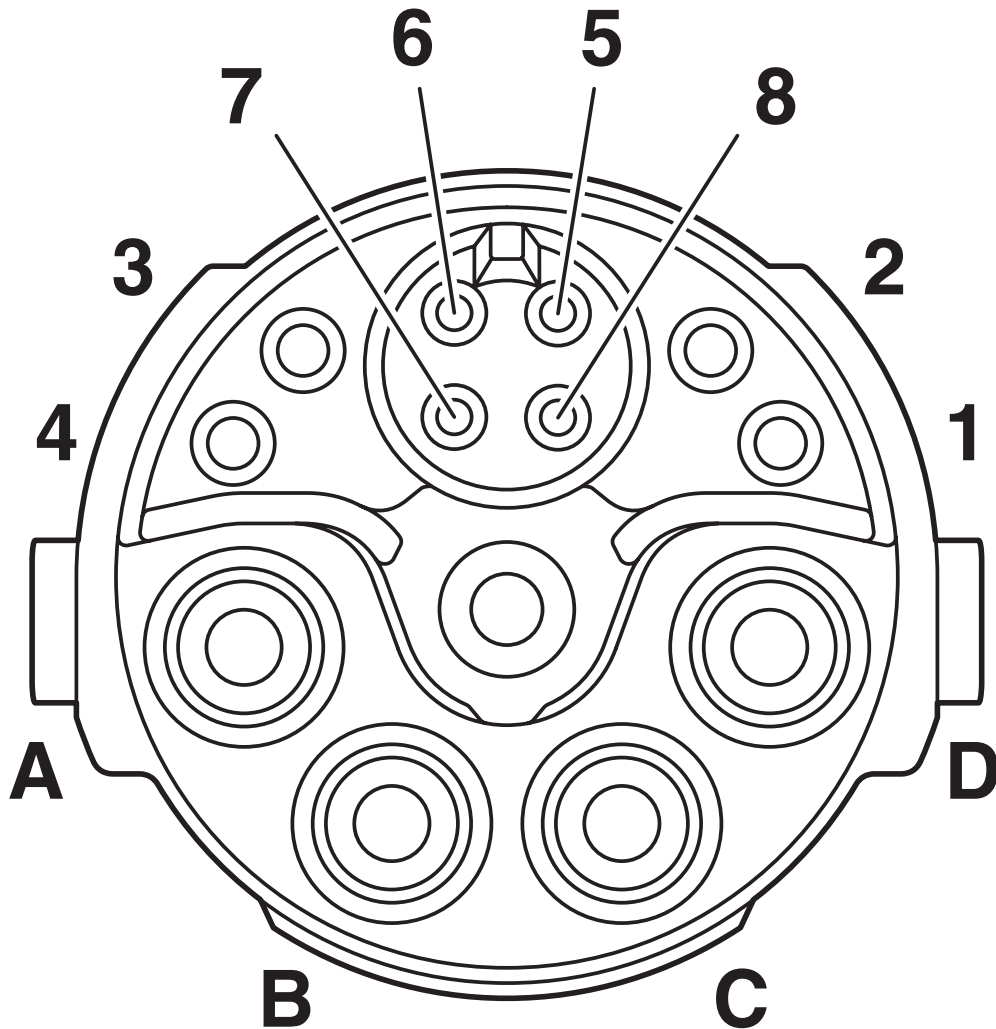
Schemazeichnung
