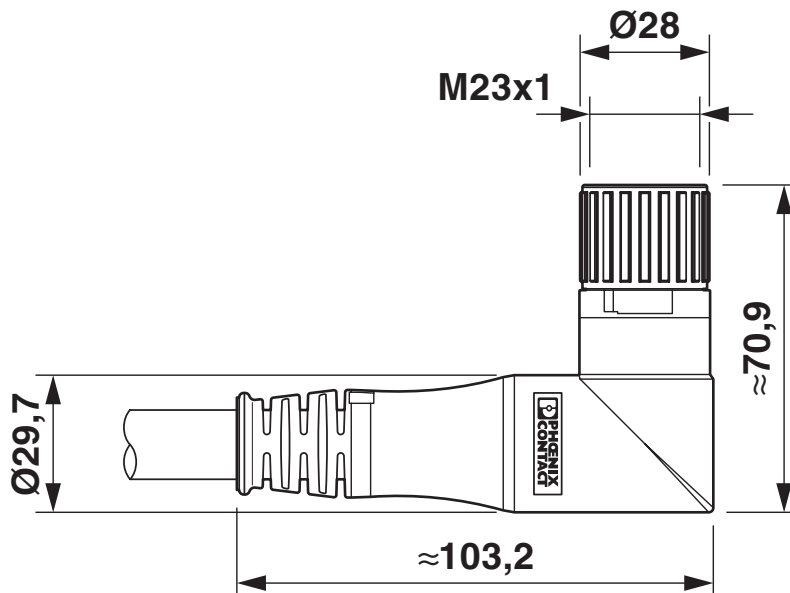
Maßzeichnung
